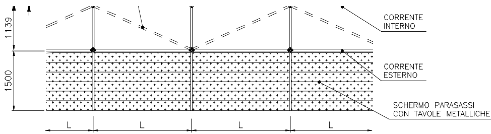
SCHEMA DI FACCIATA
