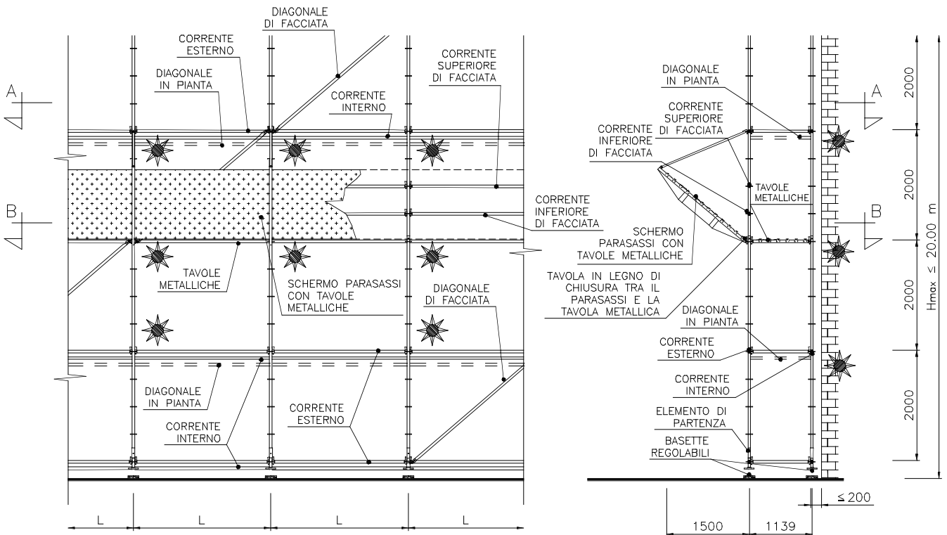
SEZIONE B-B
